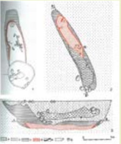
WALKOWICE, GM. CZARNKÓW, STAN. 6. RZUT POZIOMY GROBU SZKIELETOWEGO NR 1 I NR 2. LEGENDA: 1. GRÓB NR 1; 2 I 3 GRÓB NR 2 ORAZ PROFIL GROBU SZKIELETOWEGO. LEGENDA: A. SZAROBRUNATNY PIASEK; B. CIEMNOBRUNATNY PIASEK; C. JASNOSZARY PIASEK PRZEMIESZANY Z BRUNATNYM; D. BRUNATNY PIASEK; E. POZOSTAŁOŚCI ŁODZI; F. CAŁEC; G. KAMIEŃ (ZA GAJDA, 2006)
